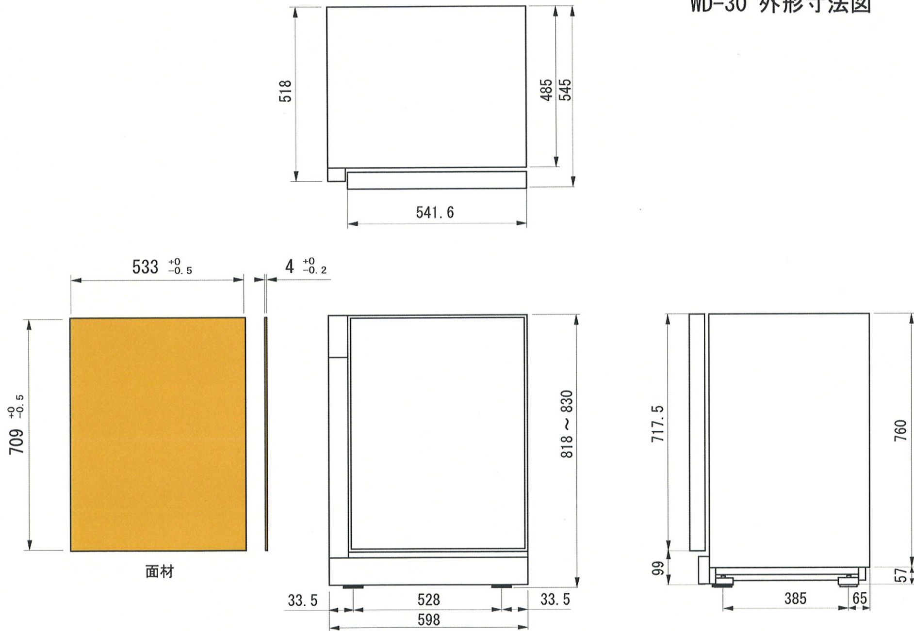
WD-30 外形寸法图
