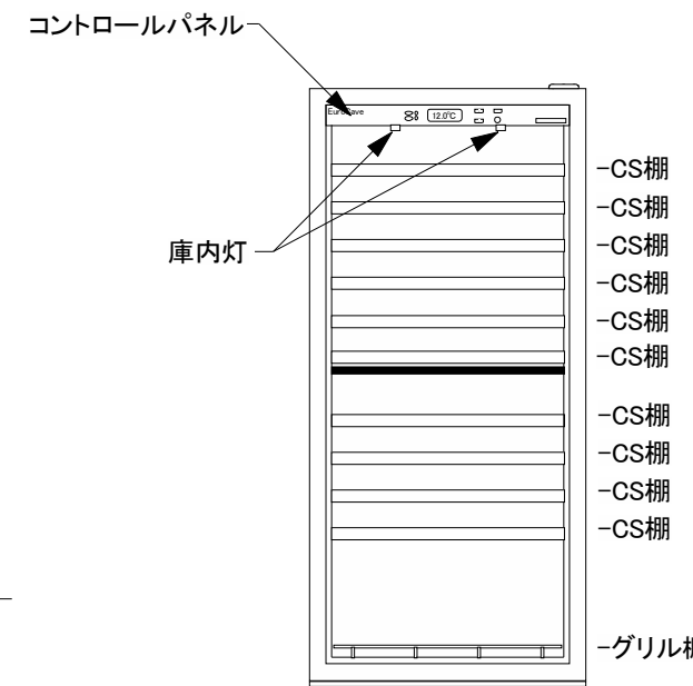
【内部正面図】
