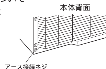
アース接続ネジ
