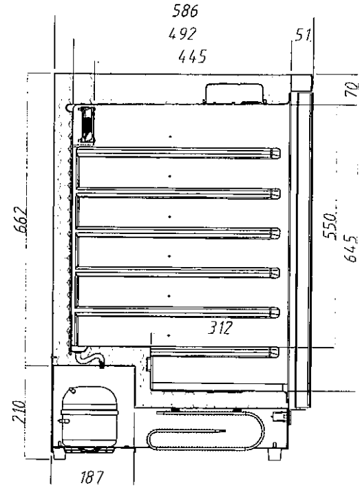
剖面 A-A
