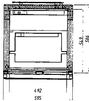
剖面 C-C
