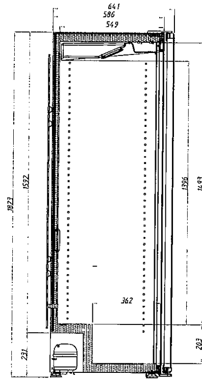
剖面 A-A
